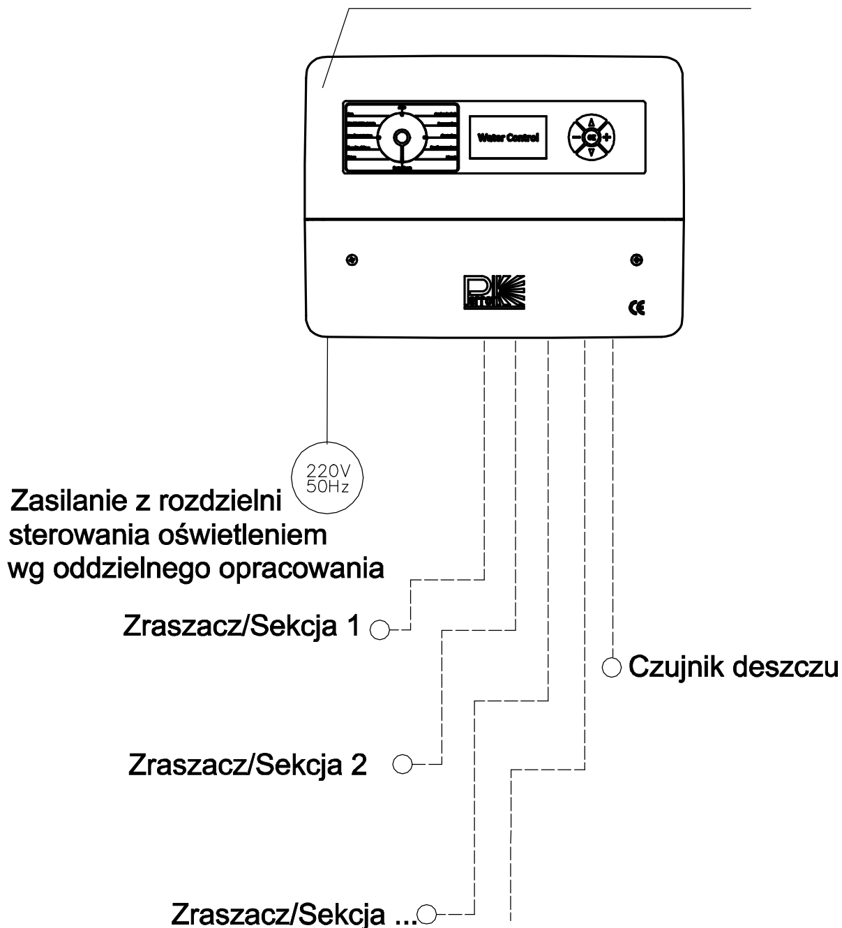
Sterownik "Water Control SC 12"
